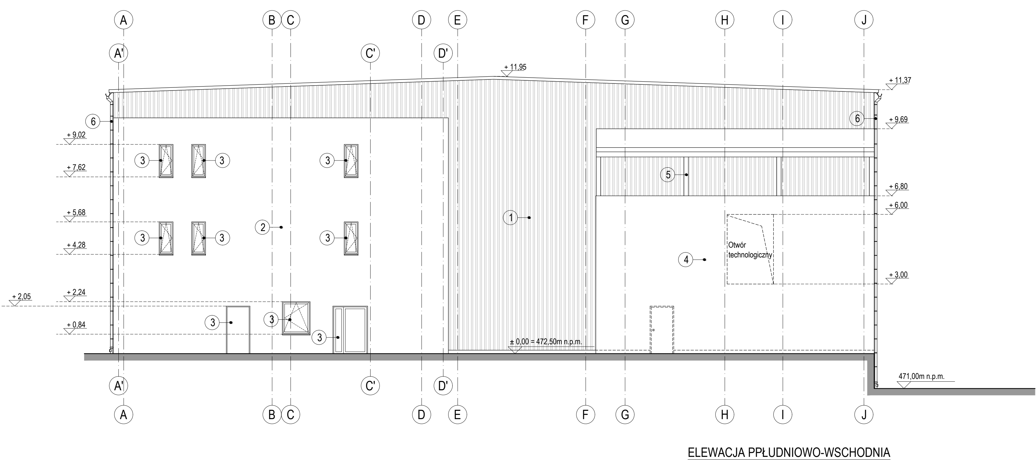
ELEWACJA PÓŁNOCNO-WSCHODNIA
