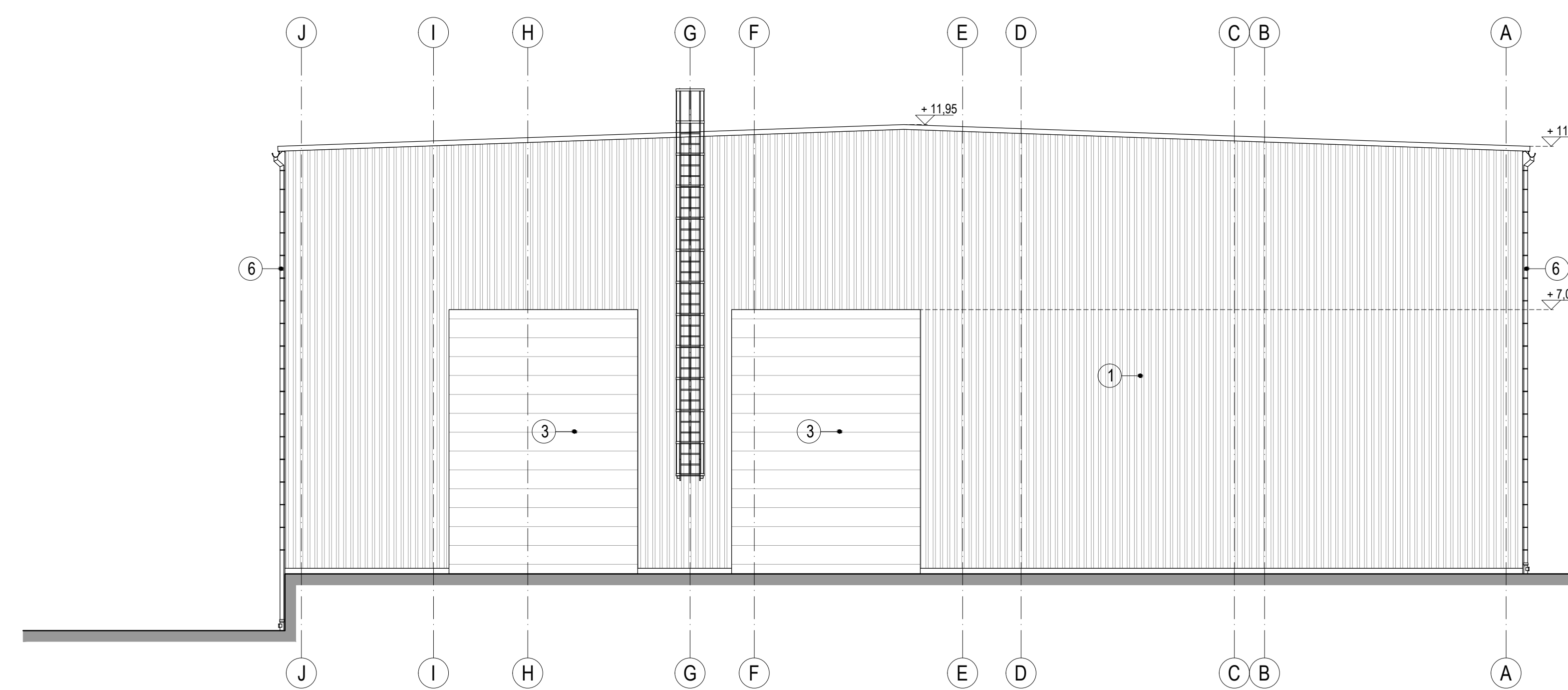
ELEWACJA PÓŁNOCNO-ZACHODNIA
